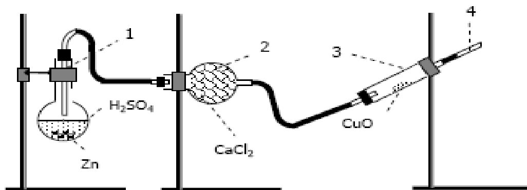
Рис.2. Установка для восстановления оксида меди(II).
